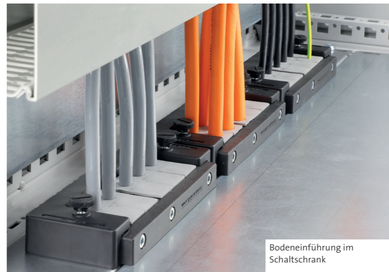
EMV Abschirmung auf Hutschiene
