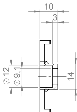
SCHNITT A-A
