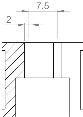
SCHNITT A-A
