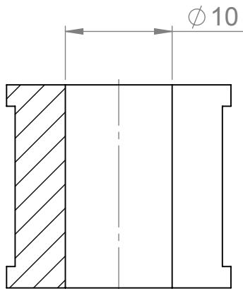
SCHNITT A-A
