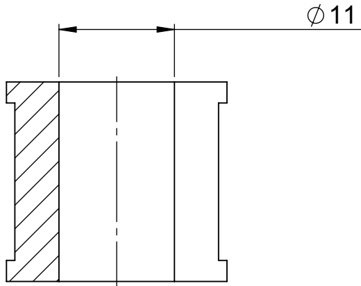
SCHNITT A-A
